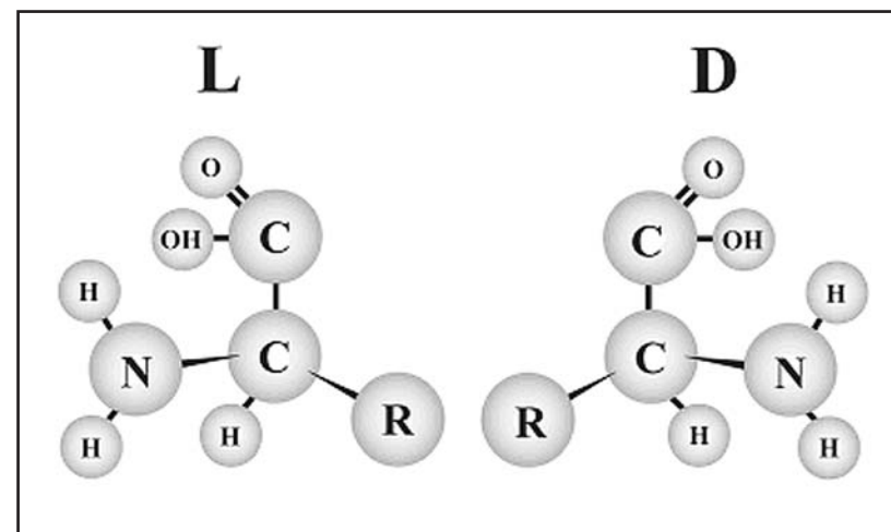
Slika 3.3. Građa D i L izomera aminokiselina. Zapazite da je raspored atoma u jednom obliku trodimenzionalna slika u ogledalu drugog. R je radikal koji znatno varira u hemijskom sastavu kod različitih vrsta aminokiselina, dok je ilustrirani deo isti za sve aminokiseline.
